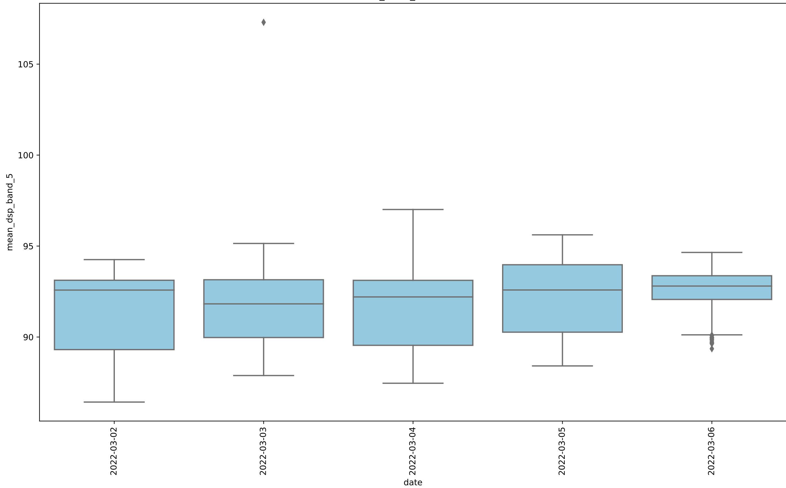
RAYOL_2022_max, band 5
