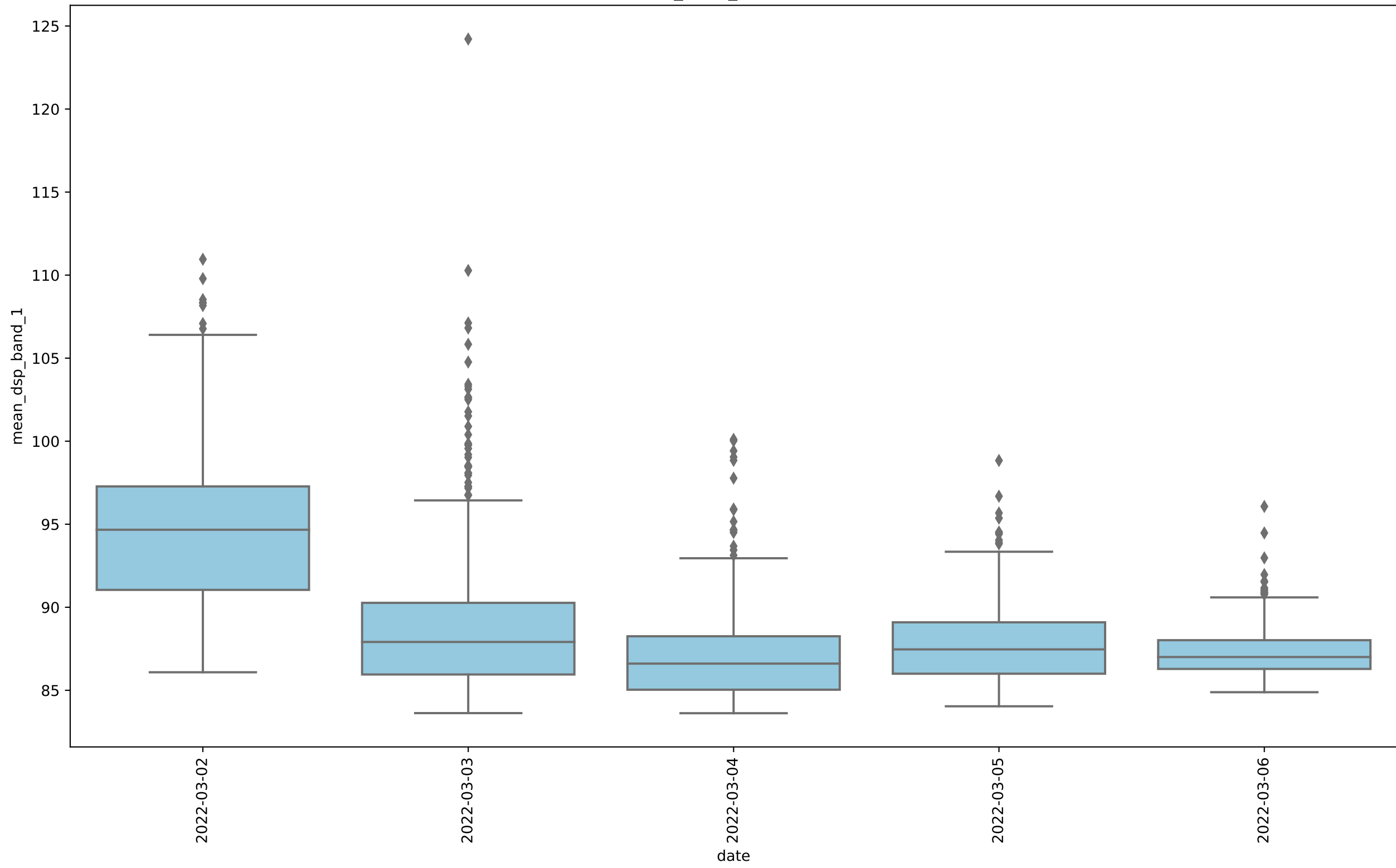
RAYOL_2022_max, band 1
