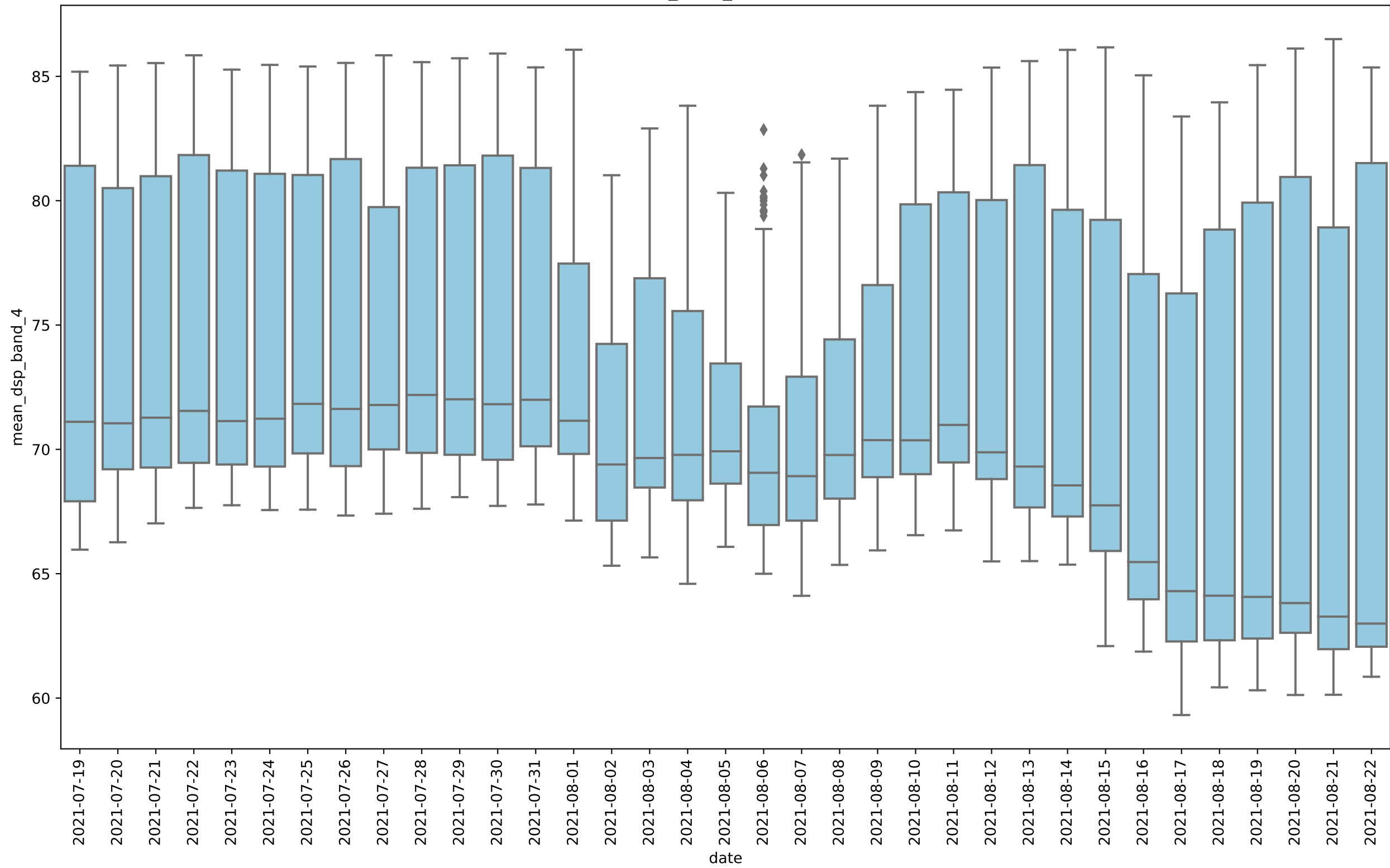
RAYOL_2021_min, band 4
