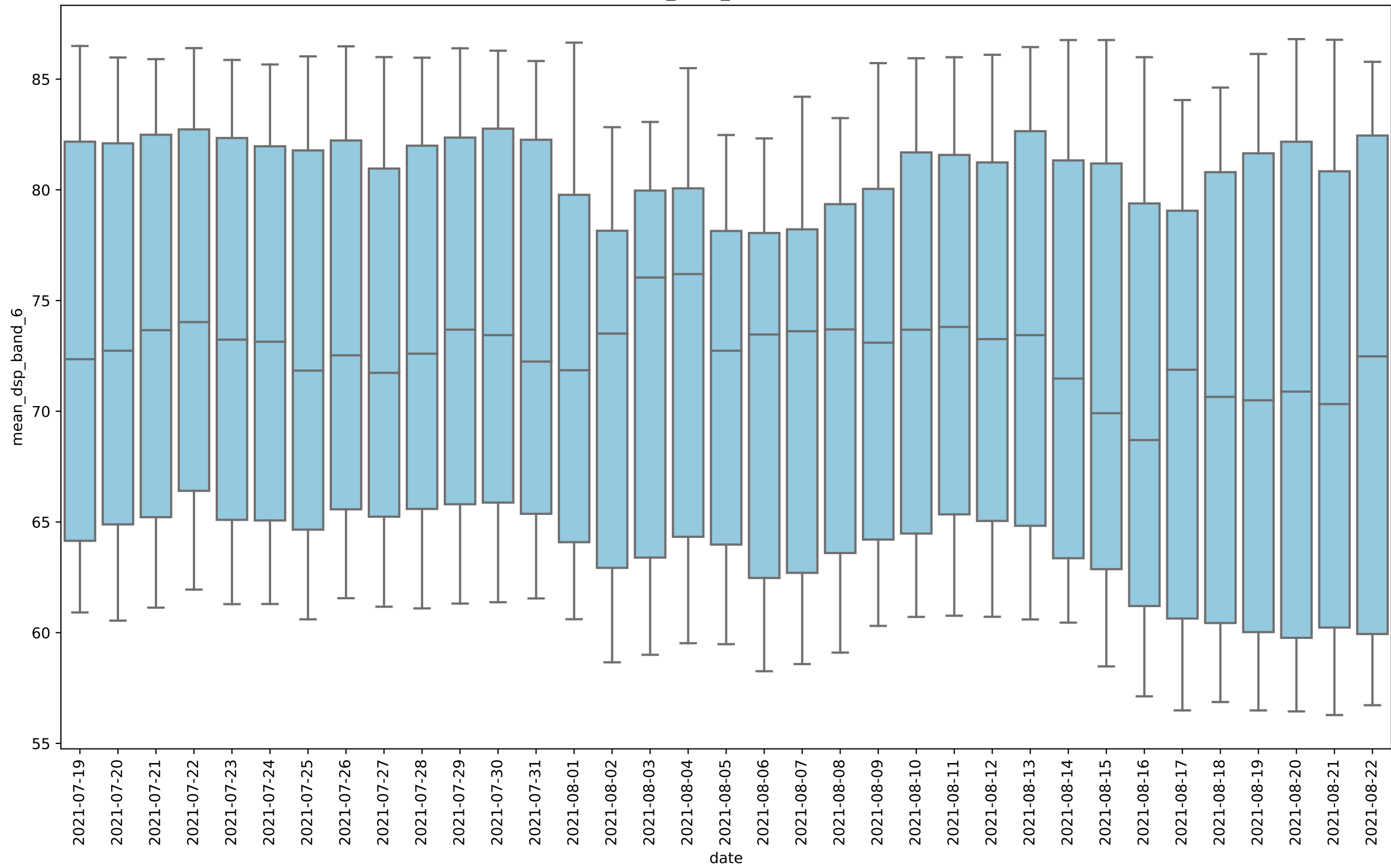
RAYOL_2021_max, band 6
