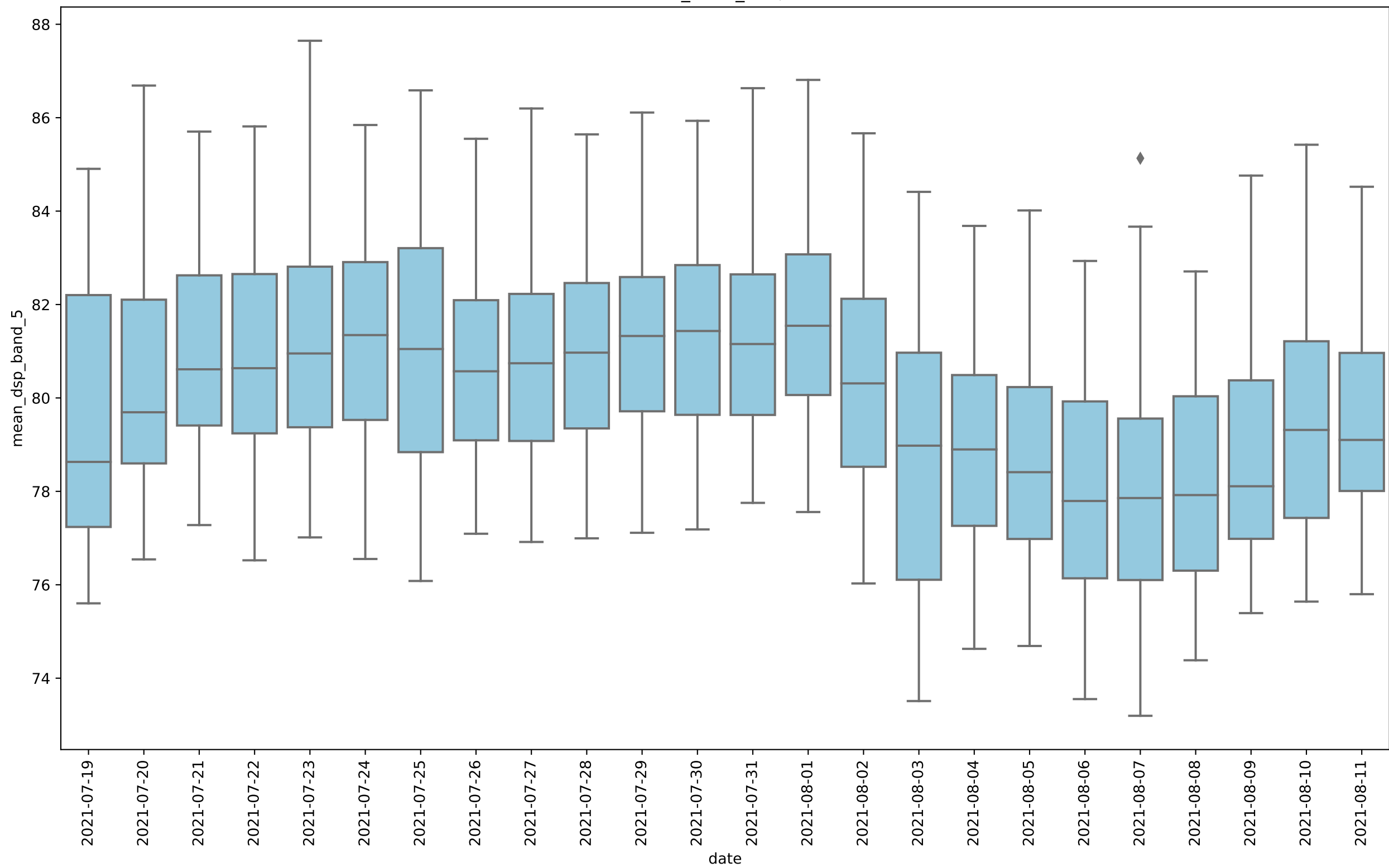
RASCASS_2021_min, band 5
